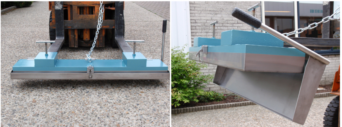
Terrainmagnet zum Einsatz auf Wegen und großen Flächen
